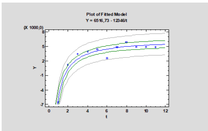
Рис. 2. Крива прогнозування
