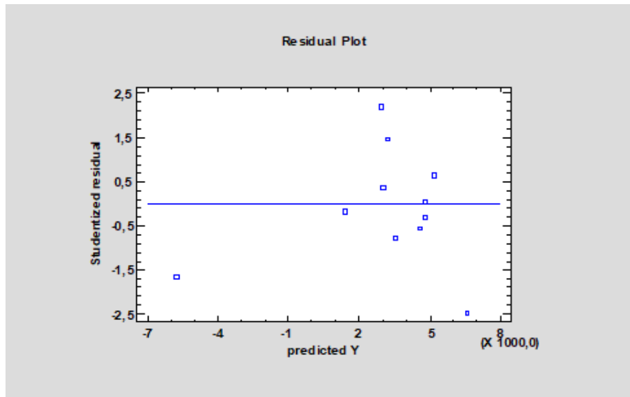
Рис. 1. Графік залишків
