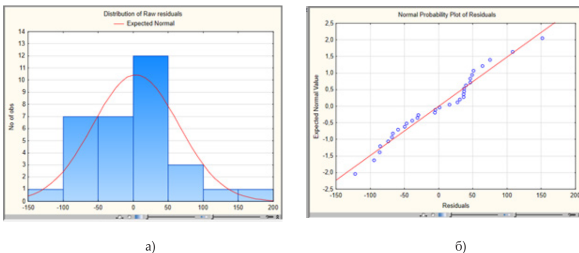
Рис. 13. Гістограма розподілу залишків моделі (а) та розподіл залишків на графіку нормального ймовірнісного розподілу (б)
